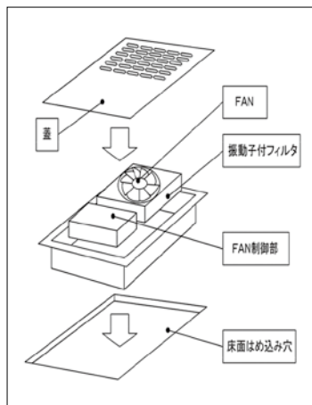
陽圧換気ユニット構成図
