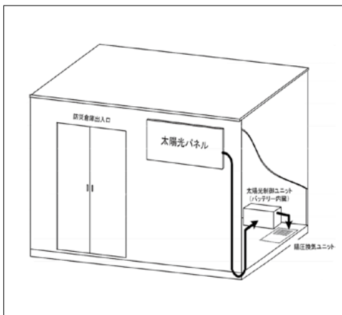
陽圧換気システム機器構成図
